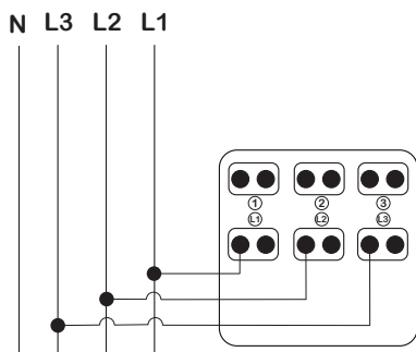
tropolna sklopka
