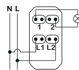
dvopolna sklopka
